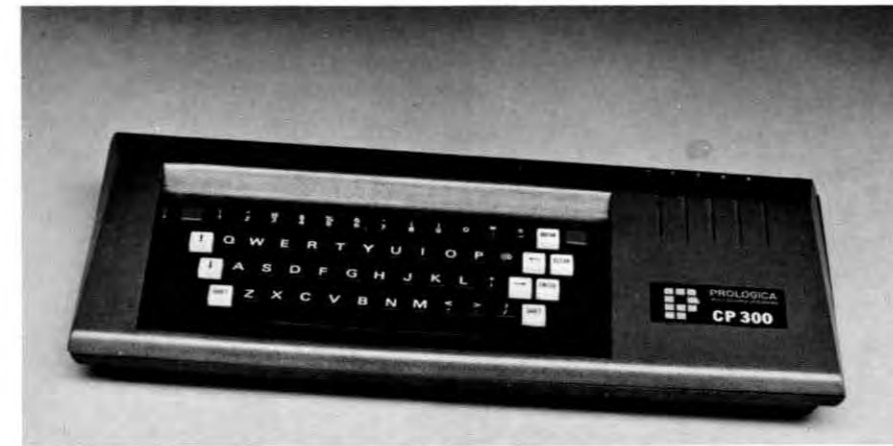
O CP-300, que em configuração básica vem com 48 Kb de RAM, teclado, conexão para vídeo e interface para cassete, pode ser ligado a drive de até quatro disquetes e impressora.
